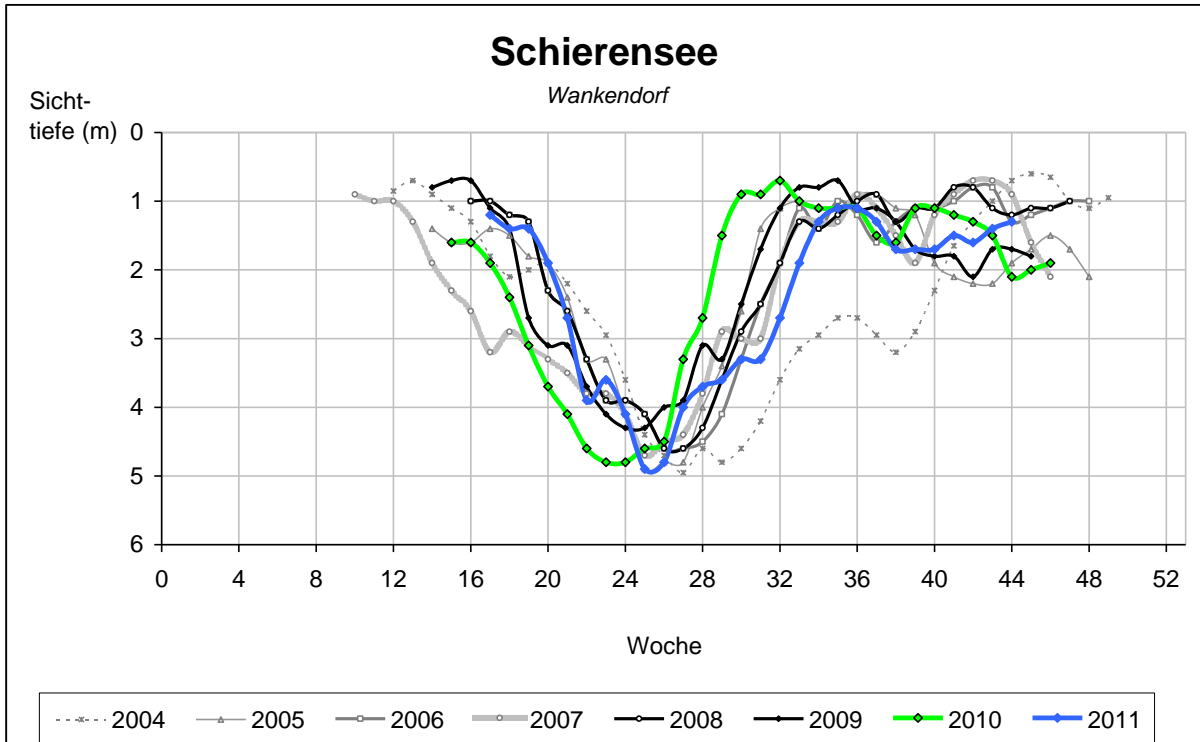
Abb.7: Saisonaler Verlauf der Sichttiefen im Jahresgang
