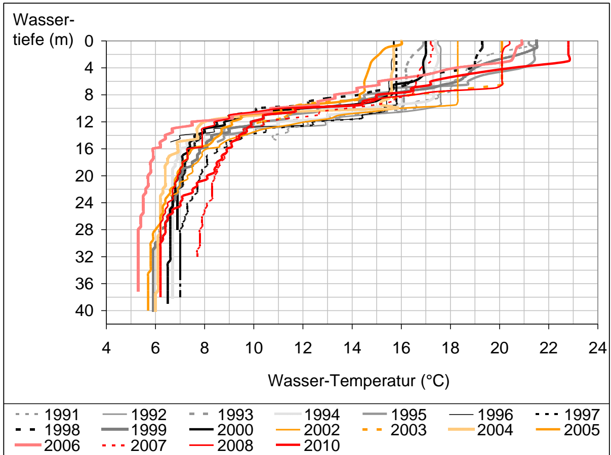
Abb.7: Vertikalprofile der Wassertemperatur im Sommer
