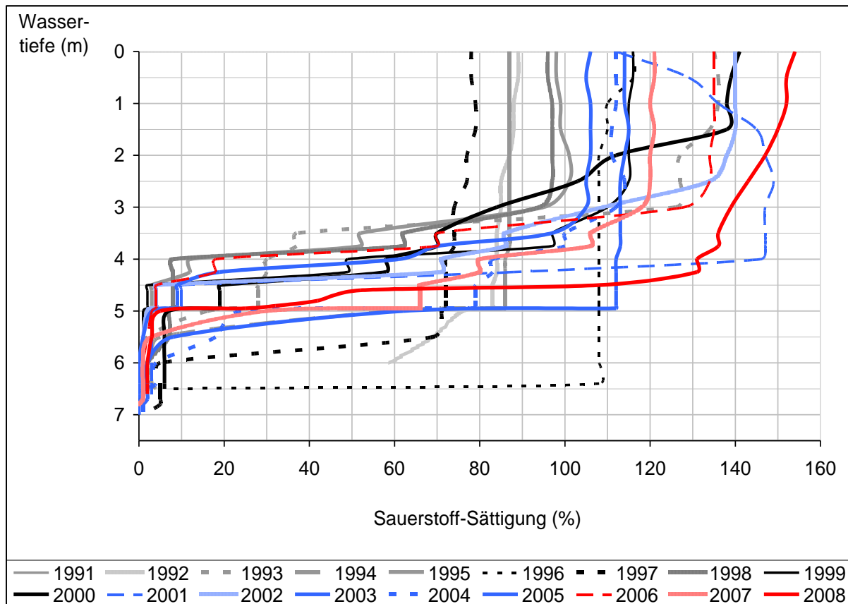
Abb.7: Vertikalprofile der Sauerstoff-Sättigung im Sommer
