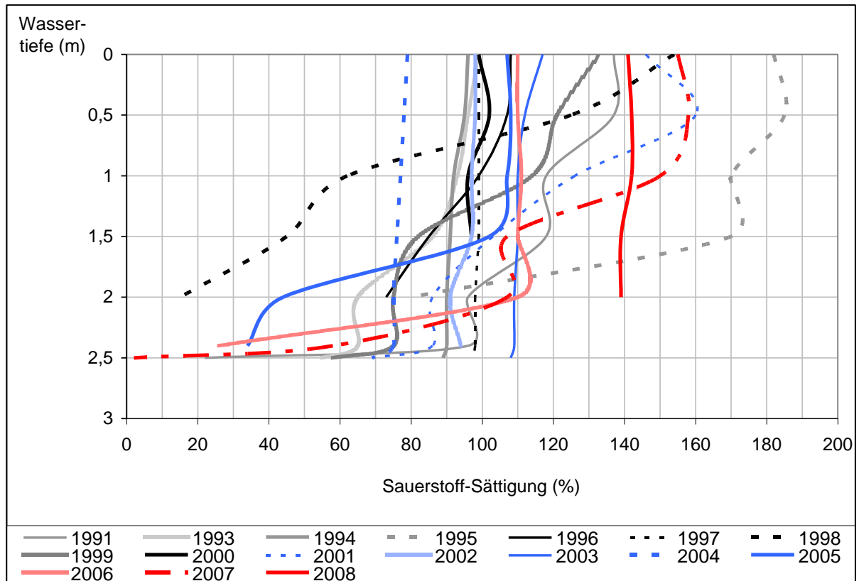
Vertikalprofile der Sauerstoff-Sättigung im Sommer
